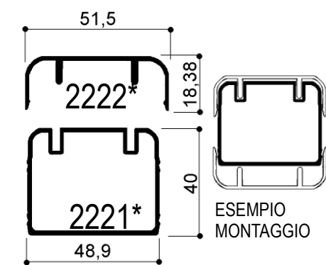
DISEGNI META' DEL VERO (1:2)- SCALE 1:2
