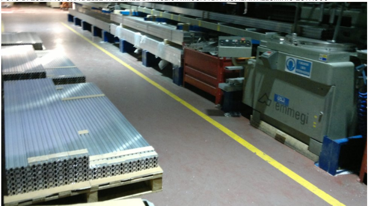
FOTO DI ESEMPIO: UNA DELLE TRE LINEE DI TAGLIO A MISURA DI PROFILI IN ALLUMINIO ESTRUSO
