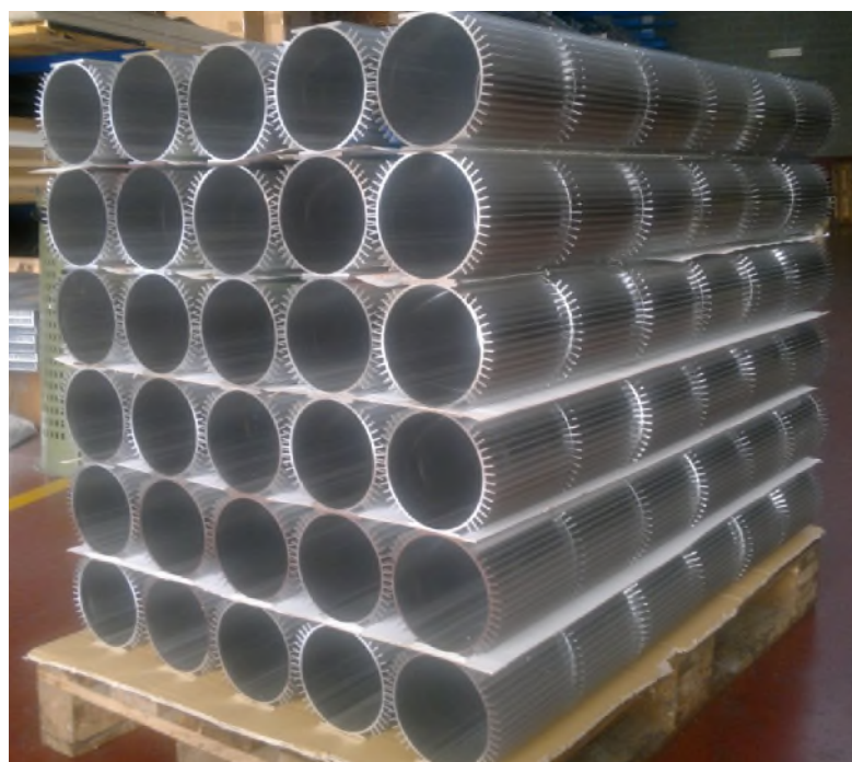
EXEMPLE DE PHOTO : PROFILÉS EN ALUMINIUM EXTRUDÉ POUR CARTERS DE MOTEUR ÉLECTRIQUE
