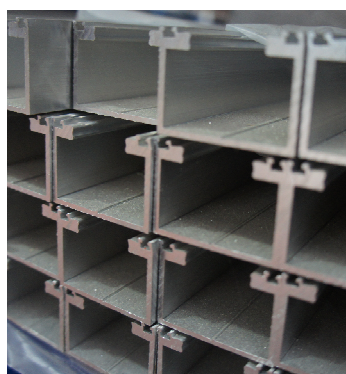
EXEMPLE DE PHOTO : DIVERS PROFILS EXTRUDÉS PERSONNALISÉS
