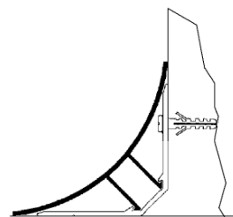
PRZYKŁAD MONTAŻ
