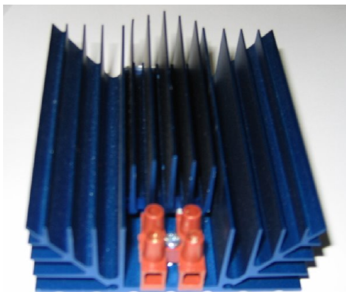
PRZYKŁADOWE ZDJĘCIE: PROFILE WYCIĄGANE I OBRÓBKOWANE DO ZASTOSOWANIA JAKO GRZEJNIKI/REZYSTORY
