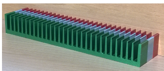
PRZYKŁADOWE ZDJĘCIE: PROFILE ALUMINIOWE WYCIĄGANE PŁASKIE RADIATORY
