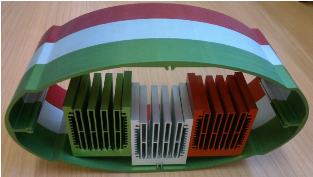
PRZYKŁADOWE ZDJĘCIE: PROFILE ALUMINIOWE WYCIĘTANE NA WYMIAR I ANODOWANE
